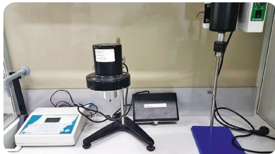
Универсальный ионметр, ротационный вискозиметр, лопастная мешалка
